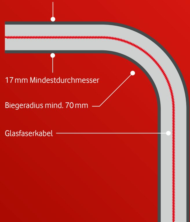
Abbildung: M25-Leerrohr
